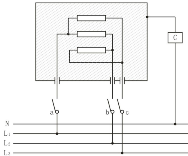
图 3 三三相连接的 II 类器具在工作温度下泄漏电流的测量电路图
